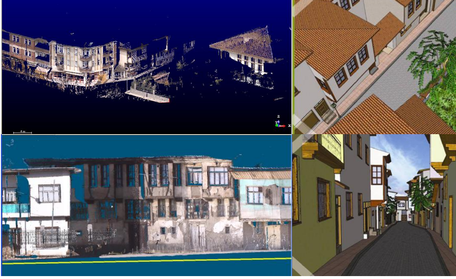
Tokat Bey Sokak Sokak Sağlıklaştırma Projesi 3D Perspektiflerinin ve Animasyonlarının Hazırlanması
